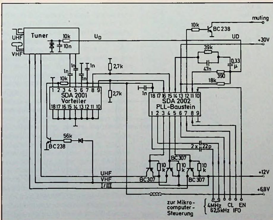
Bild 41 b: Vorteller und Phasenregelkreis des Frequenzsynthesizers SDA 200
