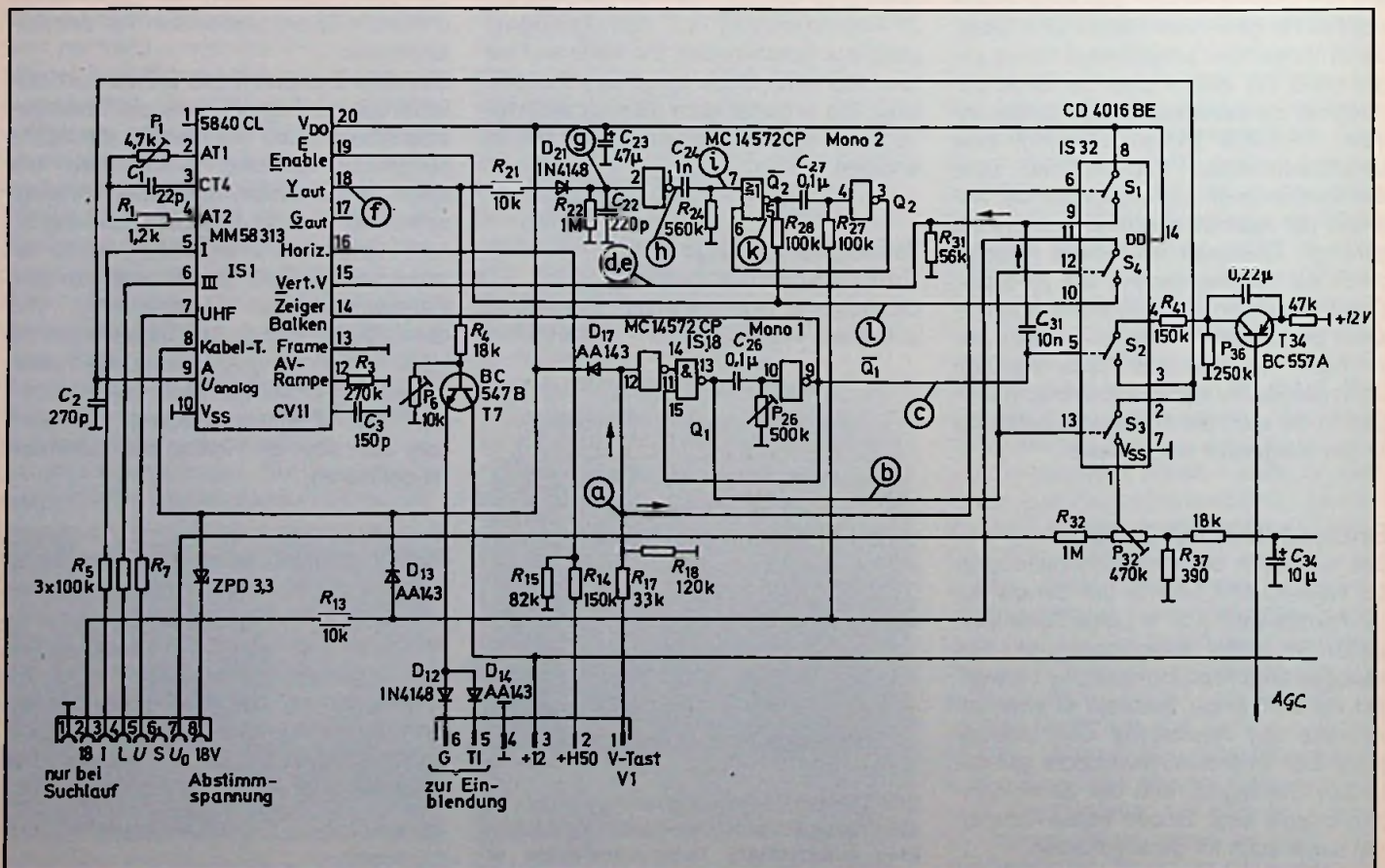
Bild 3: Schaltung des Einblend-Moduls
