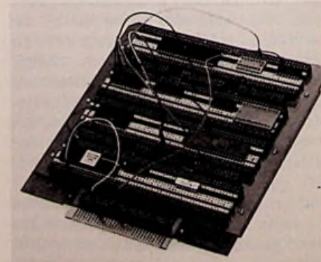
Bild 5: IC-Experimentierplatte mit DIL-Kontaktstreifen (Ouest Electronic Connecteurs)
