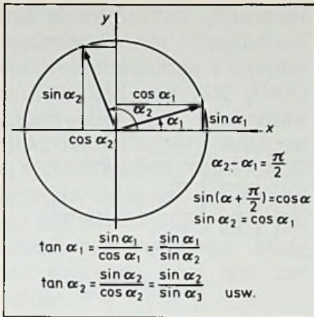
Bild 2: Erkennung des Winkels eines rotierenden Vektors durch Abtasten zu festen Zeiten
