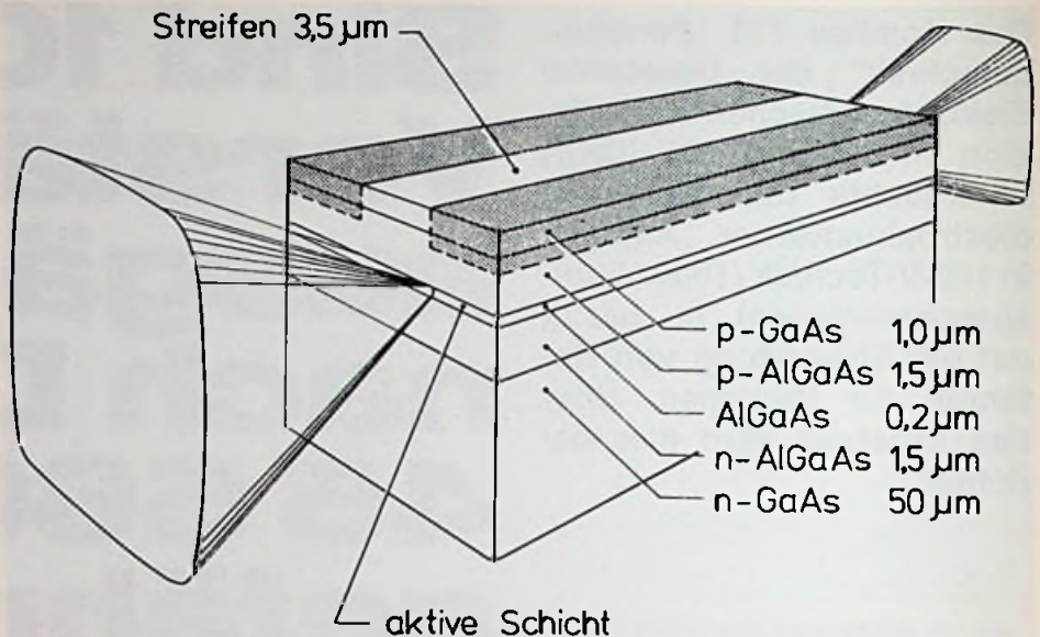
Bild 1: Schichtenaufbau des neuen Halbleiter-Lasers
