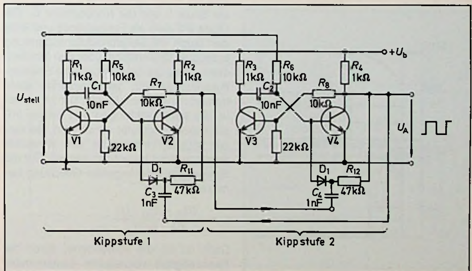
Bild 13: Monostabile Doppelkippschaltung als Impulsbreitenmodulator
