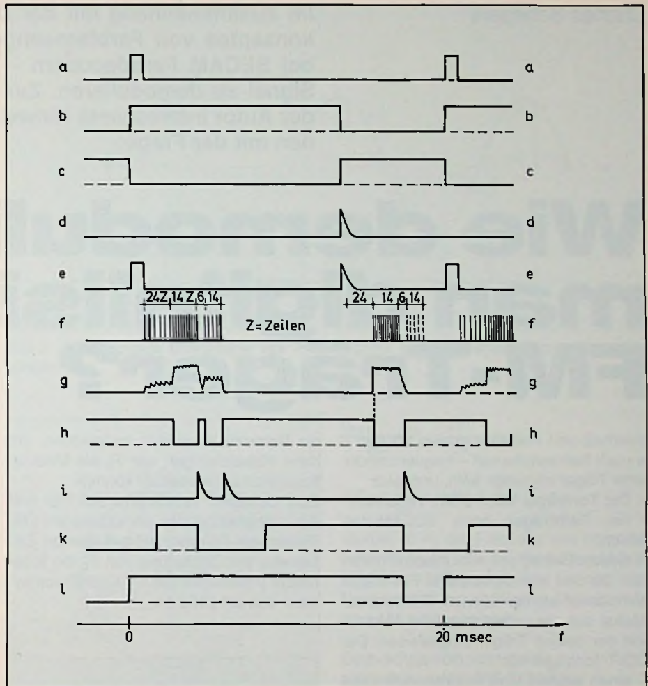
Bild 4: Impulsschema der Einblendschaltung
