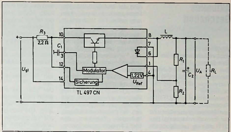
Bild 18: Schaltnetzteil mit dem Schalt-Spannungsregler TL 497 CN
