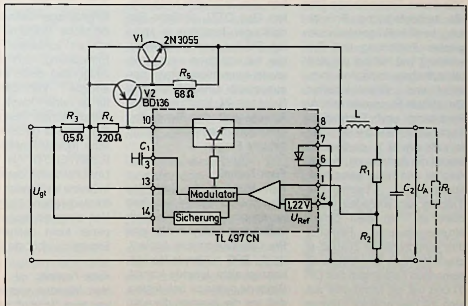
Bild 19: Schaltnetzteil mit dem Schalt-Spannungsregler TL 497 CN für größere Leistungen
