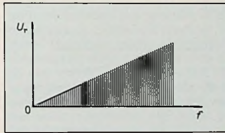
Bild 4: Dreiecksrauschen. Nach der Demodulation ergibt sich für die frequenzmäßig in Trägernähe gelegenen Rauschkomponenten ein frequenzproportionaler Amplitudenanstieg
