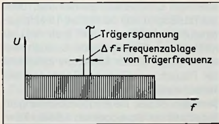
Bild 2: Spektrale Darstellung von weißem Rauschen in der Umgebung einer Trägerspannung (kontinuierliches Spektrum)
