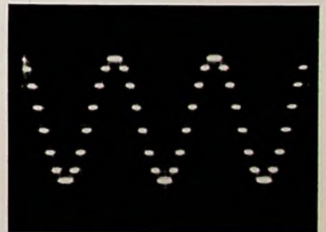
Bild 4: Aufnahme der 16stufigen Pseudo-Sinus-Schwingung
