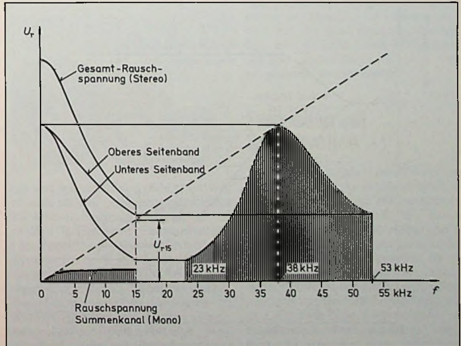
Bild 5: Auswirkungen einer Deemphase auf die Rauschspannungsanteile des Summen- und des Differenzkanals. Gesamt-Rauschspannung im Bereich 50 Hz bis 15 kHz bei Mono- und bei Stereobetrieb
