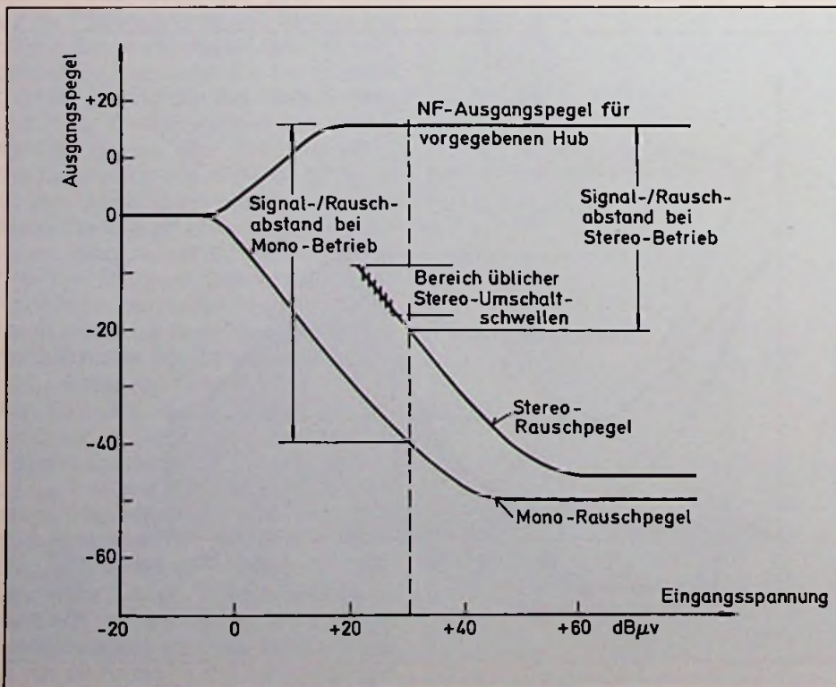
Bild 8: NF-Ausgangspegel und Rauschpegel bei Mono- und Stereobetrieb in Abhängigkeit von der Eingangsspannung. Signal-/Rauschabstand
