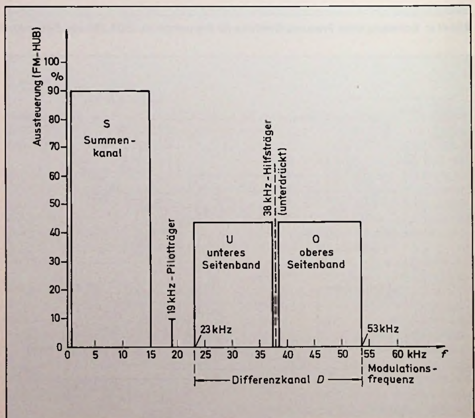
Bild 1: Aufbau des MPX-Signales, Aussteuerungsschema für UKW-FM-Rundfunksender.
