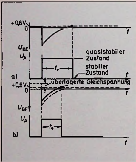
Bild 14: Basis/Emitterspannung und Ausgangsspannung einer monostabilen Klipp-schaltung
