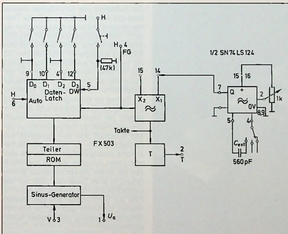
Bild 3: Detailschaltung des Sinusgenerators
