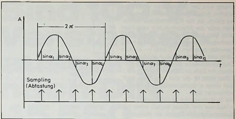
Bild 3: Zeitabhängige Darstellung des Trägersignals mit den dazugehörigen Abtastvorgängen
