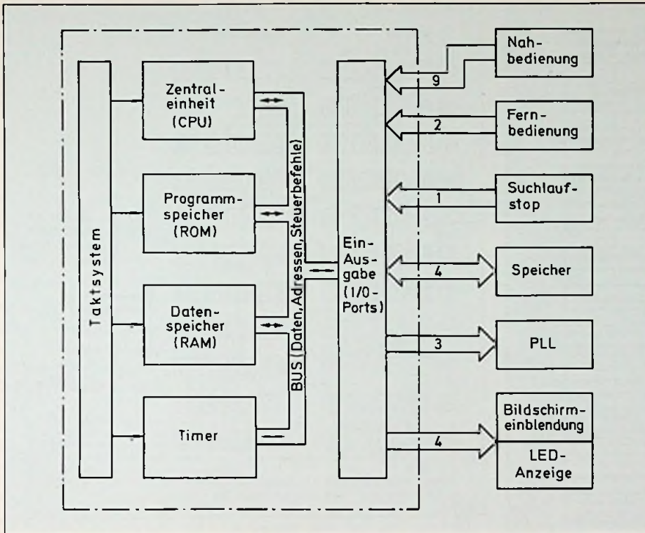
Bild 37: Blockschaltung des Mikrocomputers in Verbindung mit den Komponenten der Frequenz-Synthese
