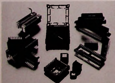
Bild 4: Auswahl an IC-Fassungen einschließlich solcher für Keramiksubstrate und Plastik-Chip-Carrier mit Kontakten an allen vier Kanten (AMP)
