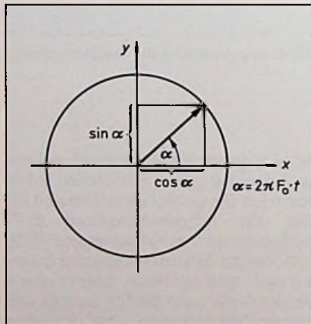
Bild 1: Darstellung eines unmodulierten Trägers als rotierender Vektor
