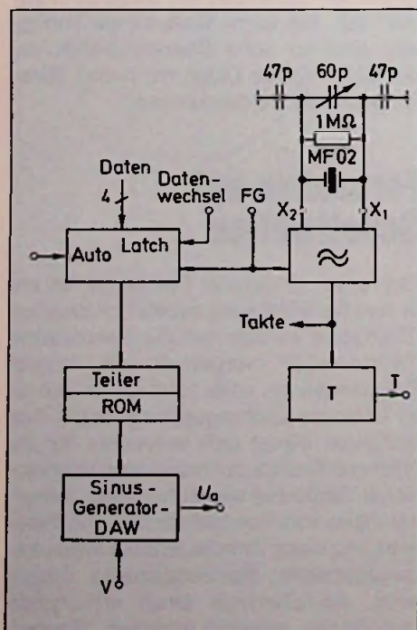
Bild 1: Prinzip des Pseudo-Sinus-Generators
