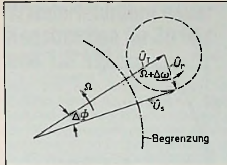
Bild 3: Das Zeigerdiagramm zeigt die Auswirkungen einer im Abstand \Delta f vom Träger gelegenen Rauschkomponente
