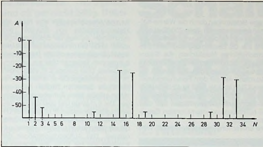
Bild 2: Spektrum des Ausgangssignals bei f_a = 1,53 \text{ kHz}
