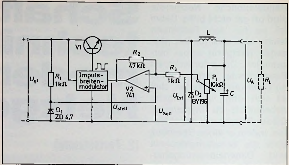
Bild 16: Grundsaltung eines einfachen Schaltnetzteiles
