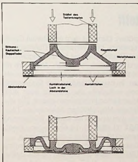
Bild 7: Funktion der Doppelfeder im Metallchassis über der Mehrlagen-Membranschaltung, oben unbetätigt, unten betätigt (Preh)
