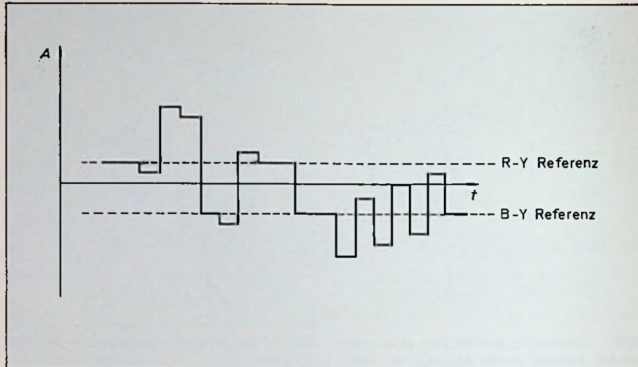
Bild 6: Ausgangsspannung des SECAM-Farbsignal-Demodulators in Abhängigkeit von der Zeit
