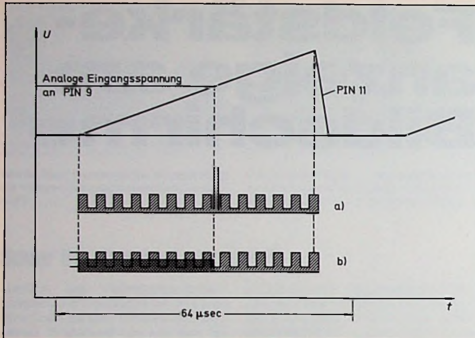
Bild 2: Das Ausgangssignal eines Vergleichers setzt den Betrag der analogen Eingangsspannung in einen schmalen Zeigerimpuls (a) oder einen längenveränderlichen Balken (b) um
