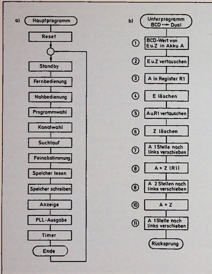
Bild 39: Softwarebeispiel als Flußdiagramm: a) Hauptprogramm, b) Unterprogramm für die BCD/Dualumwandlung
