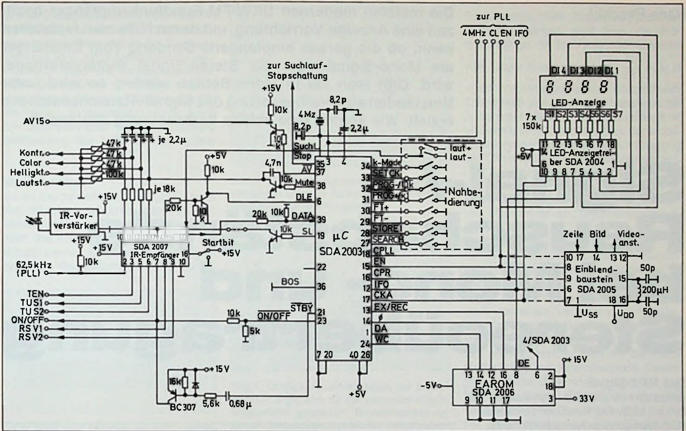
Bild 41 a: Schaltung einer Frequenz-Synthese für Fernsehgeräte (SDA 200 von Siemens); Steuerung
