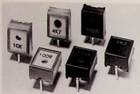
Bild 10: Gekapselte Trimpotentiometer für automatische Bestückung und automatischen Abgleich für 10 mm Raster (Valvo)
