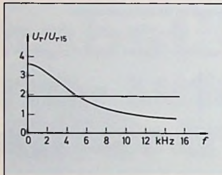
Bild 7: Aus der Gesamt-Rauschspannung ermittelter Mittelwert der Rauschspannung bei Stereobetrieb, Deemphase berücksichtigt
