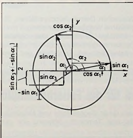
Bild 4: Vektordarstellung des frequenzmodulierten Trägersignals
