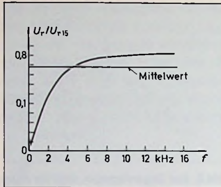
Bild 6: Aus den Rauschkomponenten des Summenkanales ermittelter Mittelwert der Rauschspannung bei Monobetrieb, Deemphase berücksichtigt
