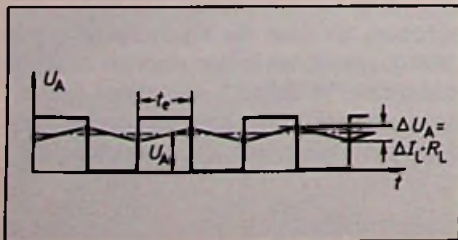
Bild 15: Durch Integration gewinnt man aus einer Pulsspannung eine Gleichspannung
